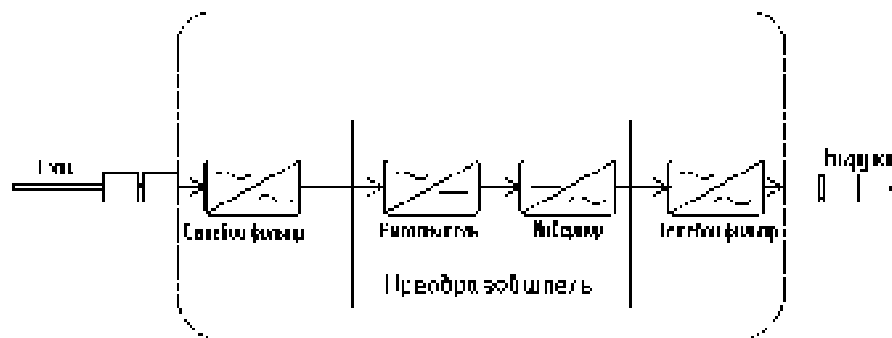
Рис. 3 – Структурная схема принципа работы стабилизаторов BAXI Energy 400 и BAXI Energy 550
